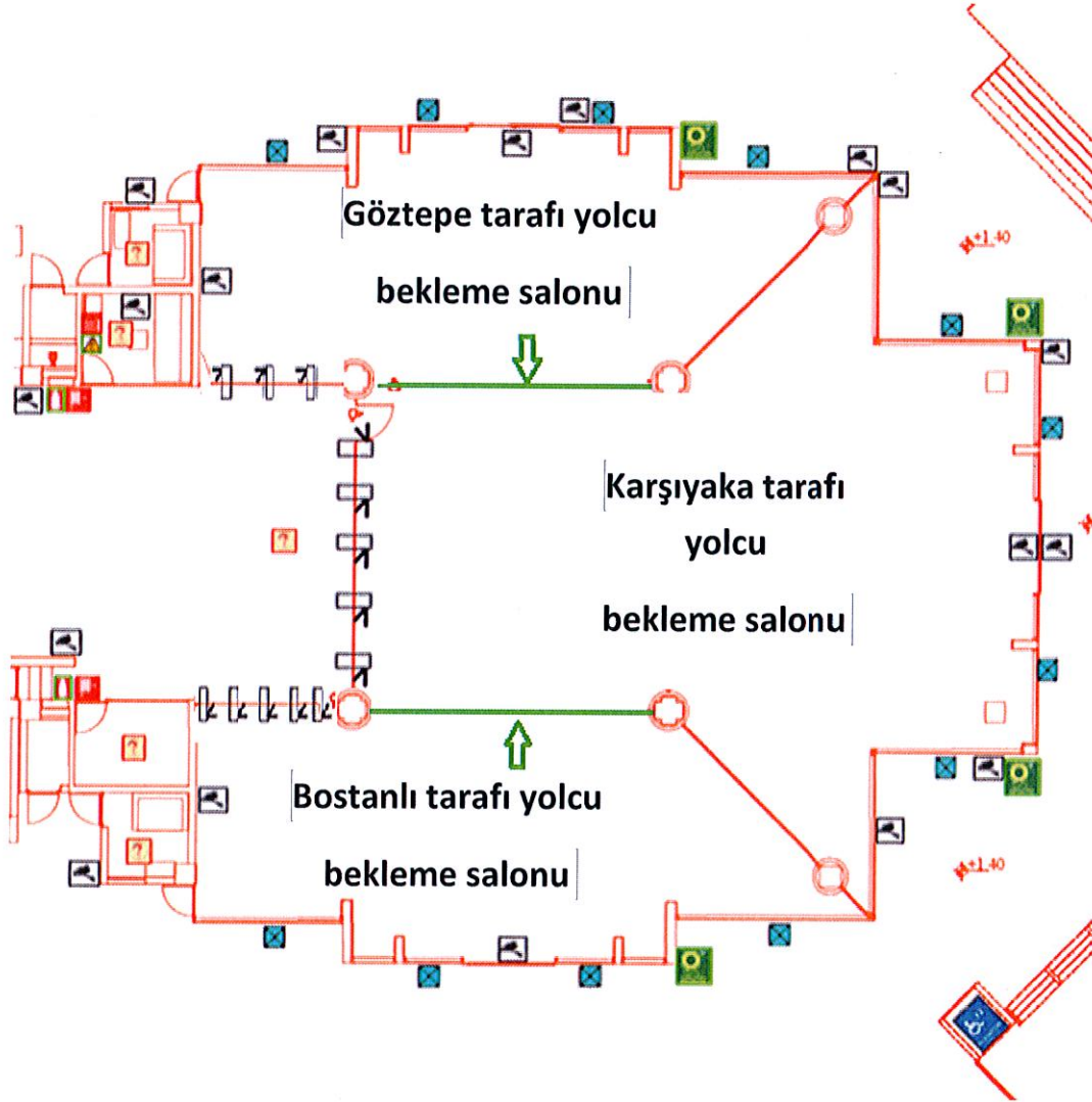
Resim 4.3. Yolcu salonunun yeniden düzenlenmesi sonucu yeni yerleşim planı
