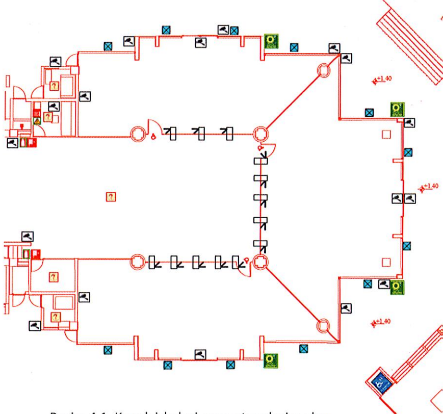
Resim 4.1. Konak iskelesi mevcut yerleşim planı
